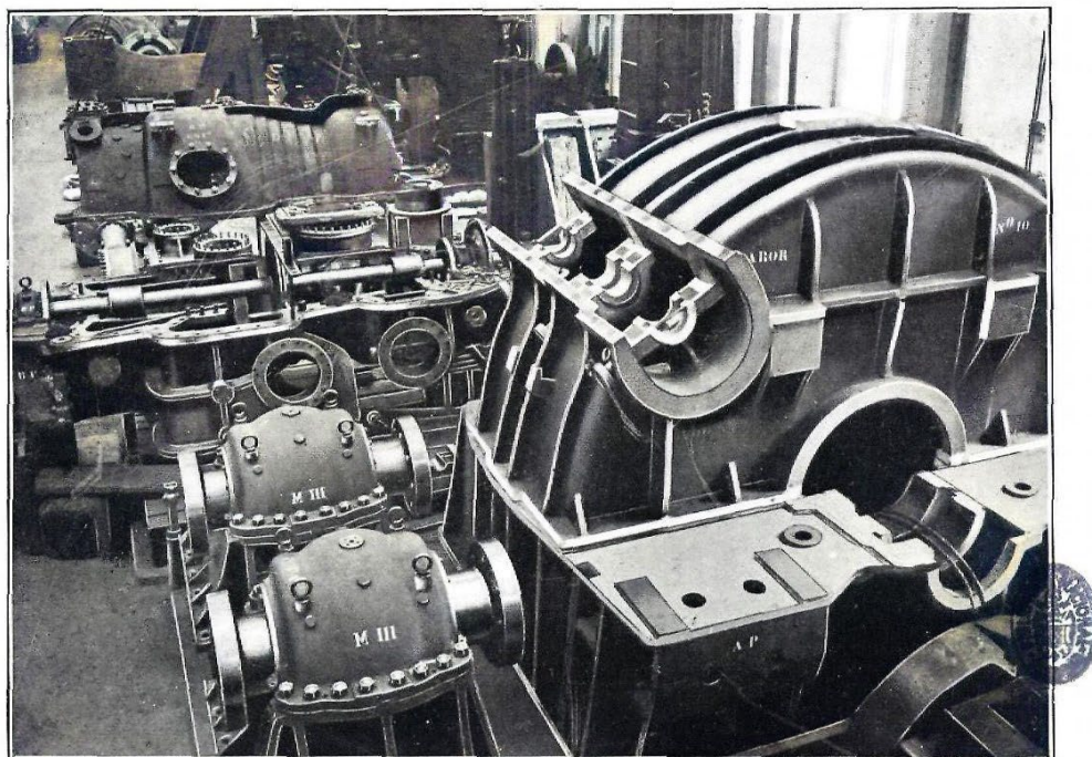
CAJA DE ENGRANAJES DE BABOR, CHUMACERAS DE EMPUJE Y TURBINA DE B. P. DE ESTIBOR PARA EL TRASATLÁNTICO "MARQUÉS DE COMILLAS".—Septiembre 1926.
